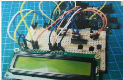
Rajah 4: Sambungan microcontroller ke LCD Display
